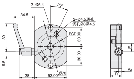
TPCC 大型位置显示器用防转动固定件
