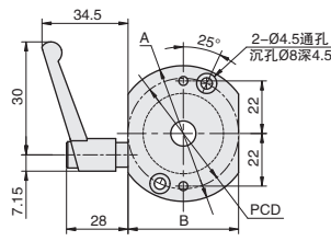
TPCB 小型位置显示器用防转动固定件
