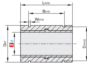
RHLPOP 开口型
