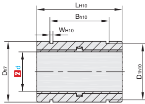
RHLP 标准型
