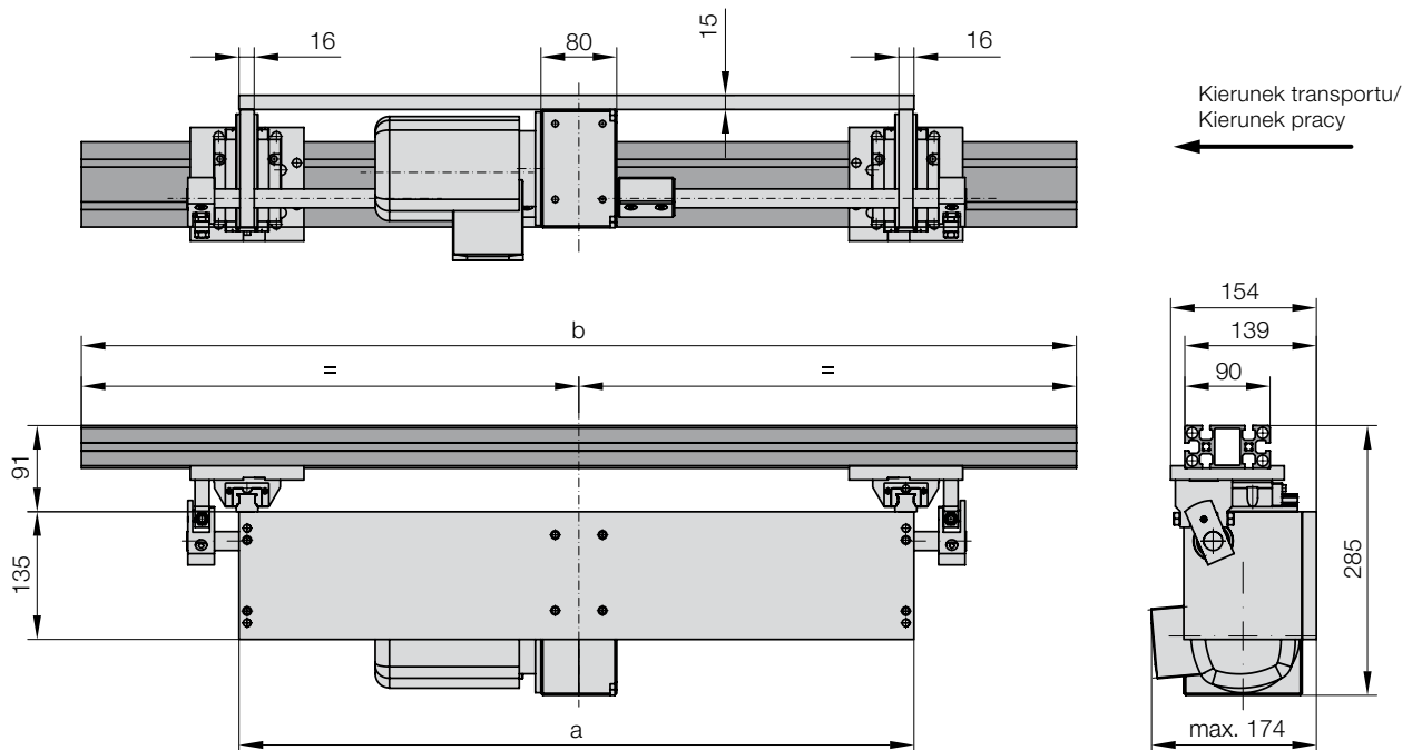
2299.221. Elektromechaniczne urządzenie transportujące, pionowe wyśrodkowane położenie przekładni, 2 szt. przewodnic, z profilem i płytą mocującą
