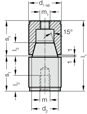
2442.12. Merkezleme ünitesi
