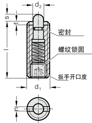
2472.07. 弹顶销, 带弹力负载销, 带有内六角头, 正常的弹力
