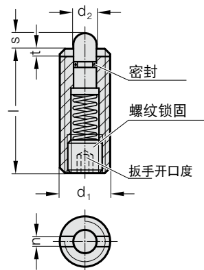
2472.37. 弹顶销, 带弹力负载销, 带有内六角头, 正常的弹力
