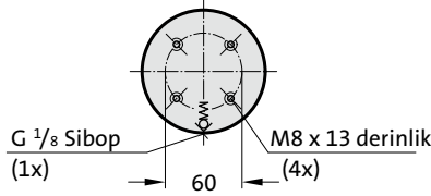
Görünüm X – Gazlı Yay
