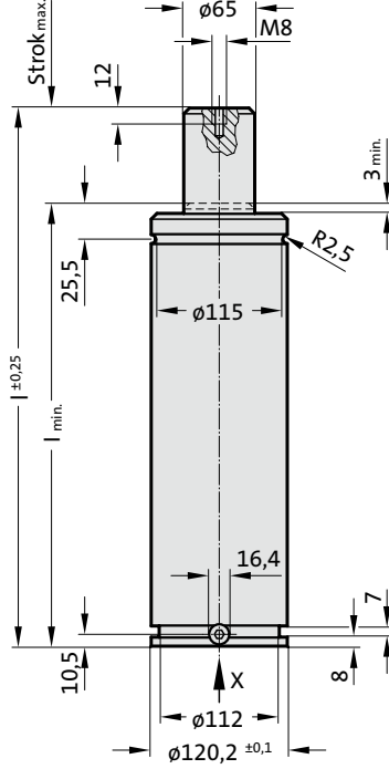
Görünüm X – Gazlı Yay
