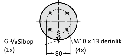
Görünüm X – Gazlı Yay
