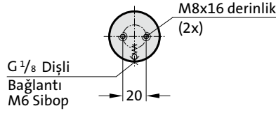
Görünüm X
