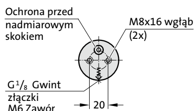
Widok X
