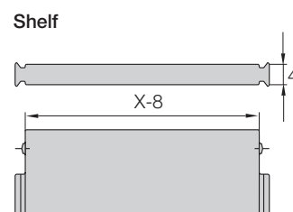
Shelf 386.X
