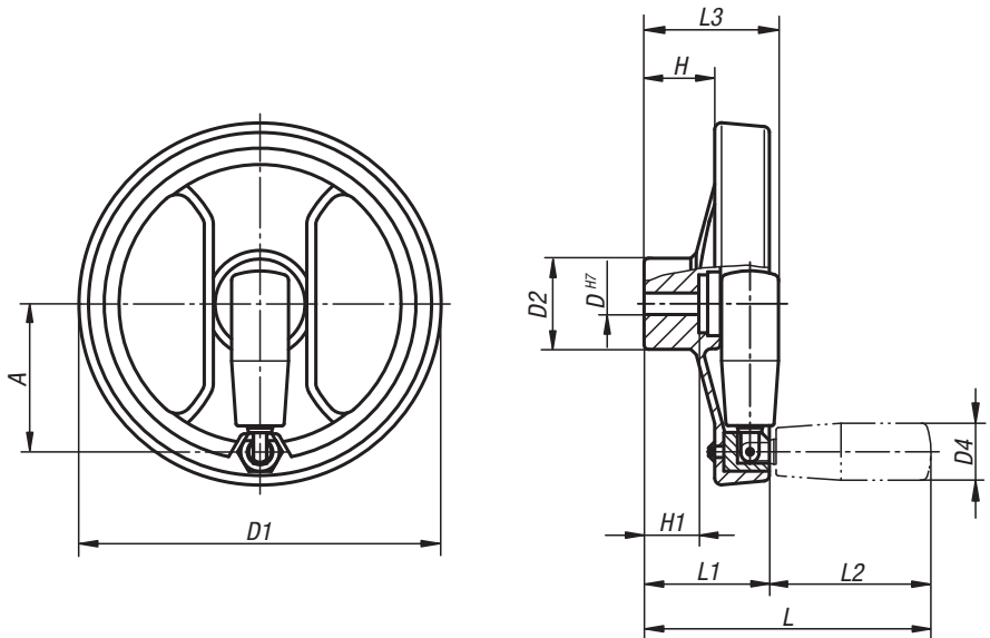
Passfedernut nach DIN 6885-1
