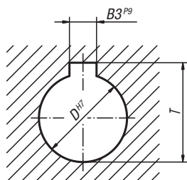
Passfedernut nach DIN 6885-1
