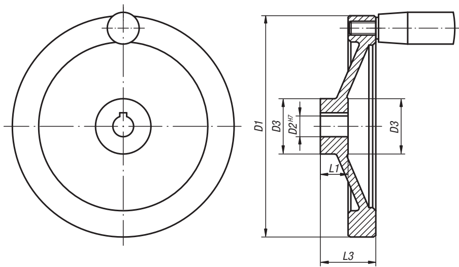
Passfedernut nach DIN 6885-1
