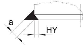
Abb. 4: Schweißnahtanordnung
