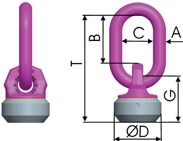
Abb. 6: Bemäßung VWBS
